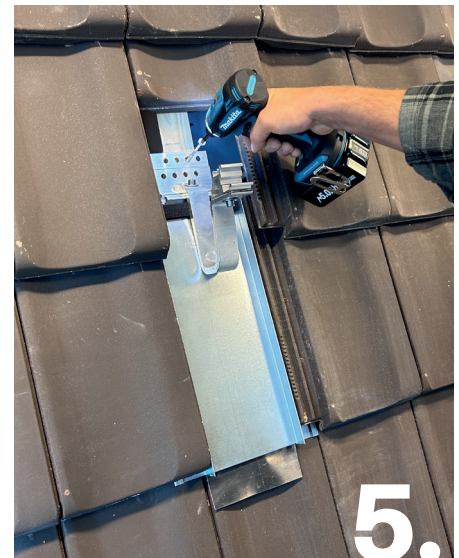
5. Dachhaken montieren.
