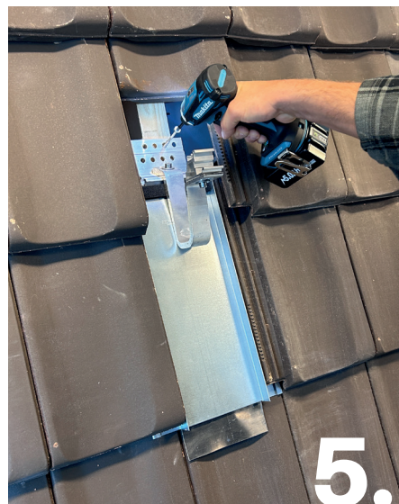
5. Dachhaken montieren.
