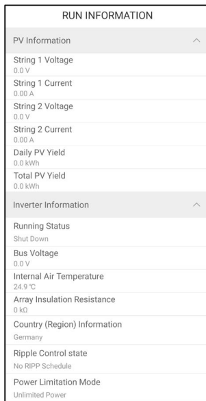
Abbildung 8-10 Betriebsdaten
