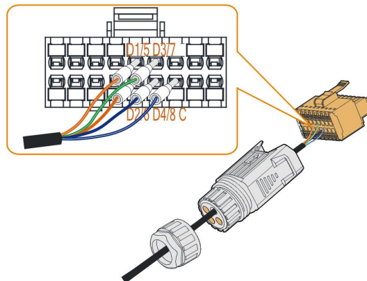
Abbildung 5-10 DI-Verbindung
