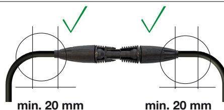
Korrekte Leitungsführung Proper cable routing
