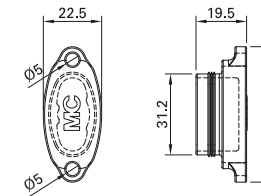
PV-SVK-EVO AC
