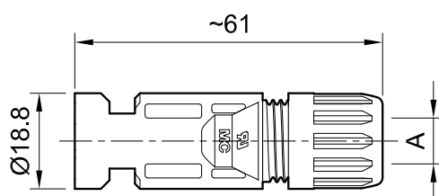
Kupplungsstecker PV-KST4...
