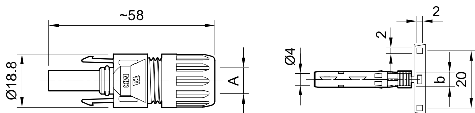
Kupplungsbuchse PV-KBT4...
