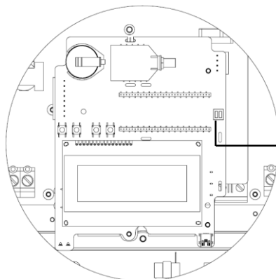
Abbildung 24: RS485 DIP-Schalter
