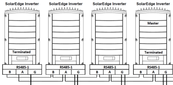
Abbildung 23: Anschluss der Wechselrichter in einem Bus
