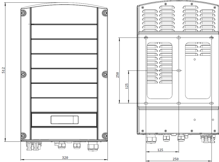
Abbildung 28: Dreiphasen-Wechselrichter mit Typ 1 Halterung - Vorder- und Rückansicht
