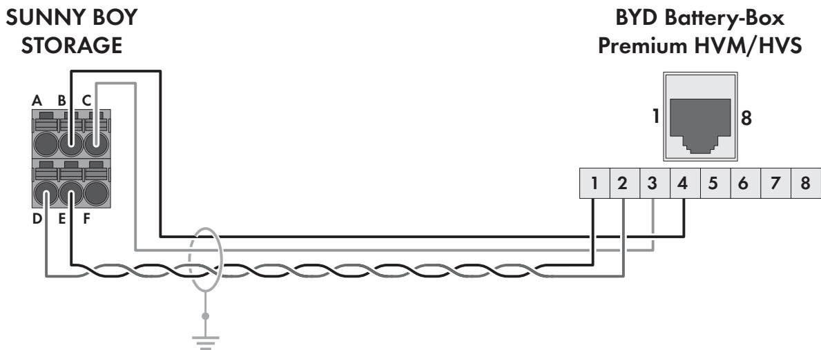
Abbildung 7: Verkabelungsprinzip SBS3.7-10 / SBS5.0-10 / SBS6.0-10 mit Battery-Box Premium HVS und HVM
