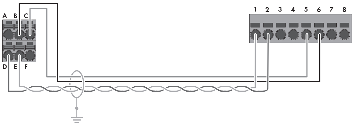
Abbildung 8: Verkabelungsprinzip SBS3.7-10 / SBS5.0-10 / SBS6.0-10 mit BMZ Hyperion, IBC era:powerbase und Axitec AXIstorage Li SH
