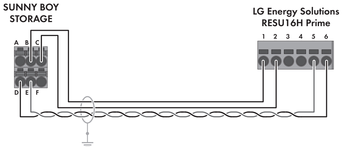
Abbildung 5: Verkabelungsprinzip SBS3.7-10 / SBS5.0-10 / SBS6.0-10 mit RESU 16H Prime
