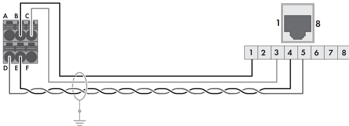
Abbildung 9: Verkabelungsprinzip SBS3.7-10 mit RESU10M
