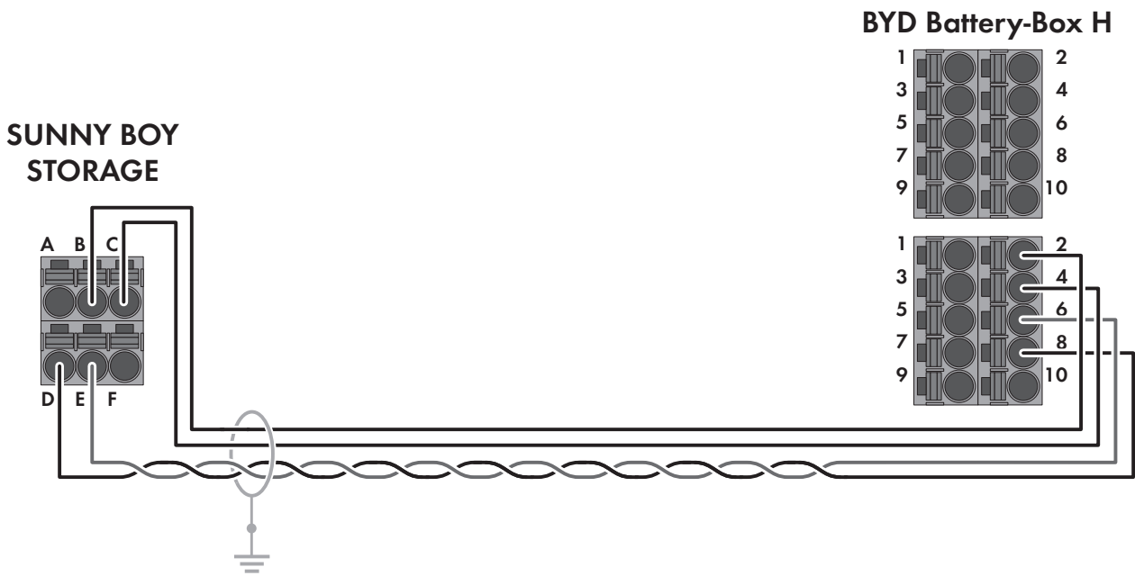
Abbildung 6: Verkabelungsprinzip SBS3.7-10 / SBS5.0-10 / SBS6.0-10 mit Battery-Box H
