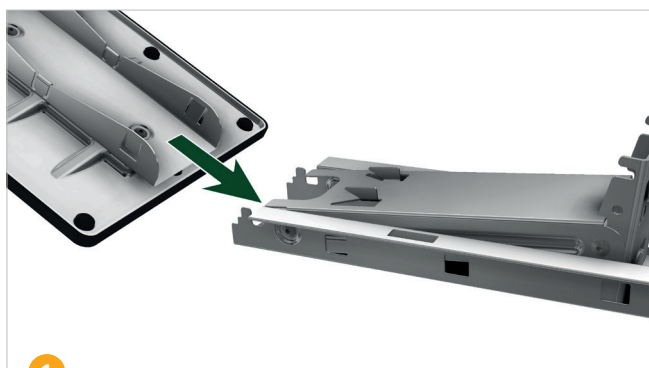
1 Bodenschuh in Führung von Basic Frame stecken.
