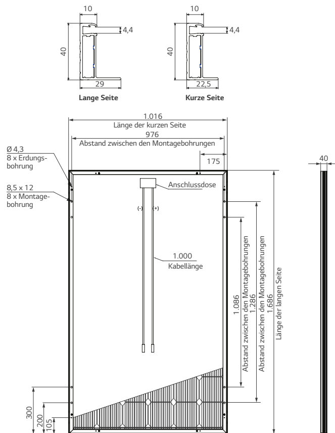
Der Abstand gilt zwischen den Mittelpunkten der Montage- und Erdungsbohrungen.
