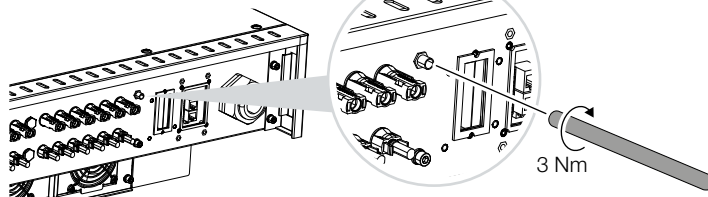
PIKO CI 50/60
