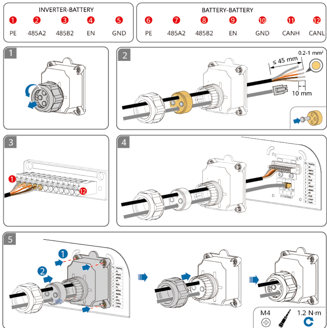
Abbildung 5-7 Signalanschlussverbindungen
