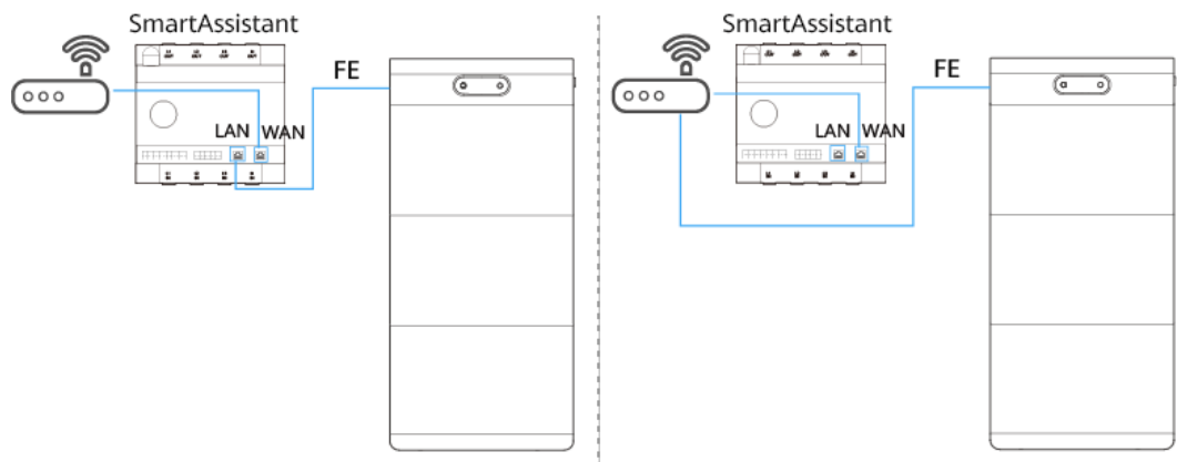
Abbildung 2-9 Netzwerkanchluss mit dem SmartAssistant oder dem Router verbunden
