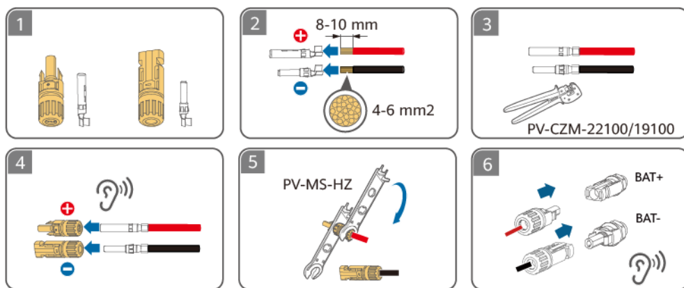
Abbildung 5-4 Anschließen der DC-Eingangstromkabel
