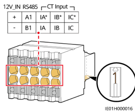
Abbildung 5-5 10-poliger Stecker
