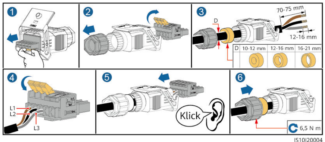
Abbildung 5-5 Dreifach adriertes Kabel (L1, L2 und L3)
