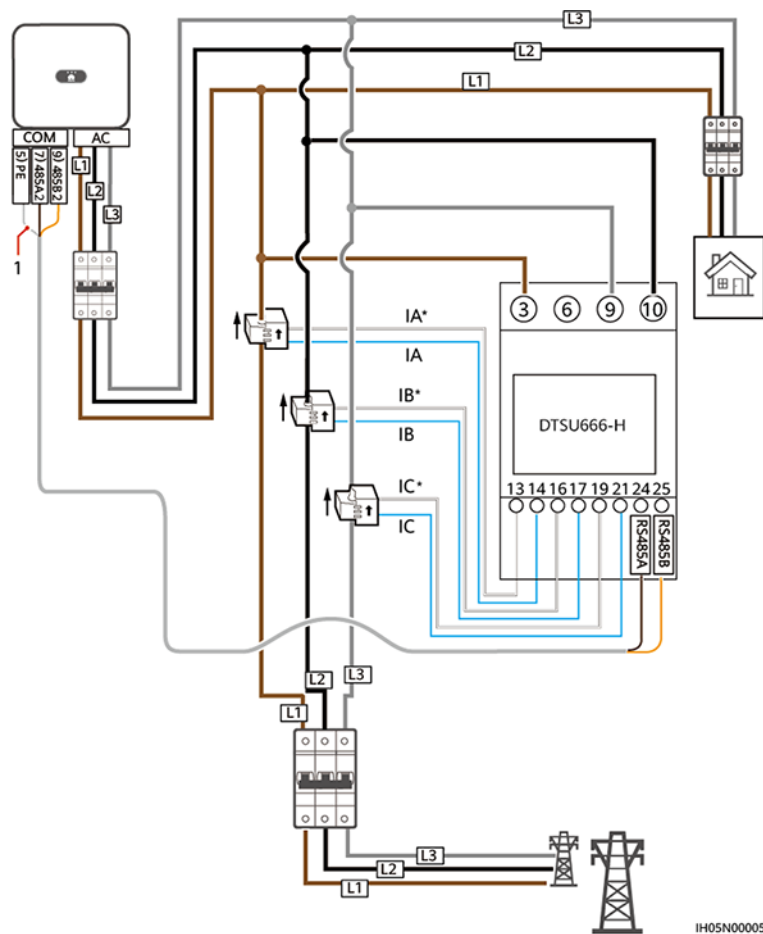
Abbildung 5-23 Dreiphasige, dreidrigige Kabelverbindung mit DTSU666-H (Smart Dongle-Vernetzung)
