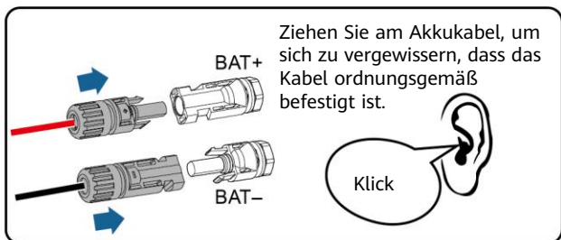
Akkuklemmen (BAT+/BAT-)
