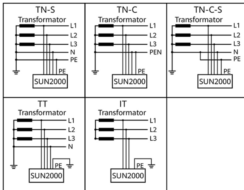
Abbildung 2-3 Stromnetze
