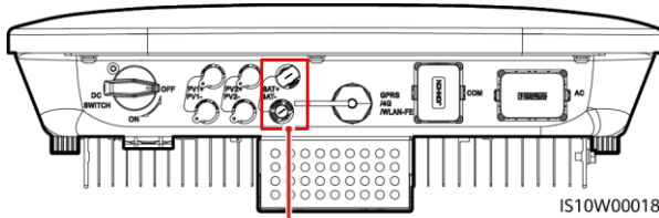
Akkuklemmen (BAT+/BAT-)
