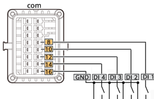
Abbildung 5-39 Kabelverbindung
