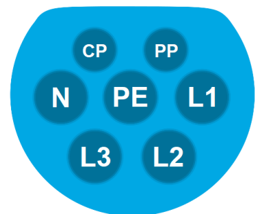
Abbildung 4: Typ 2 Stecker weiblich
