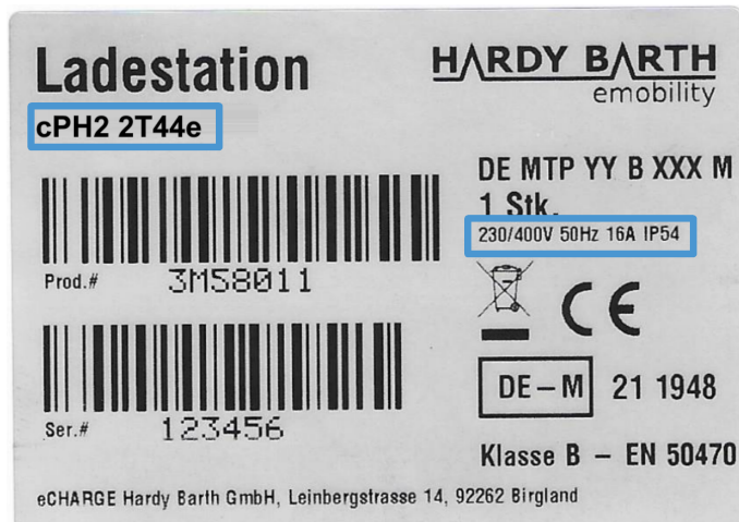
Abbildung 1: Typenschild cPH2
