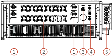
GW75K-HT/GW80K-HT/GW100K-HT Unterseite
