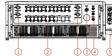
GW75K-HT/GW80K-HT/GW100K-HT Unterseite
