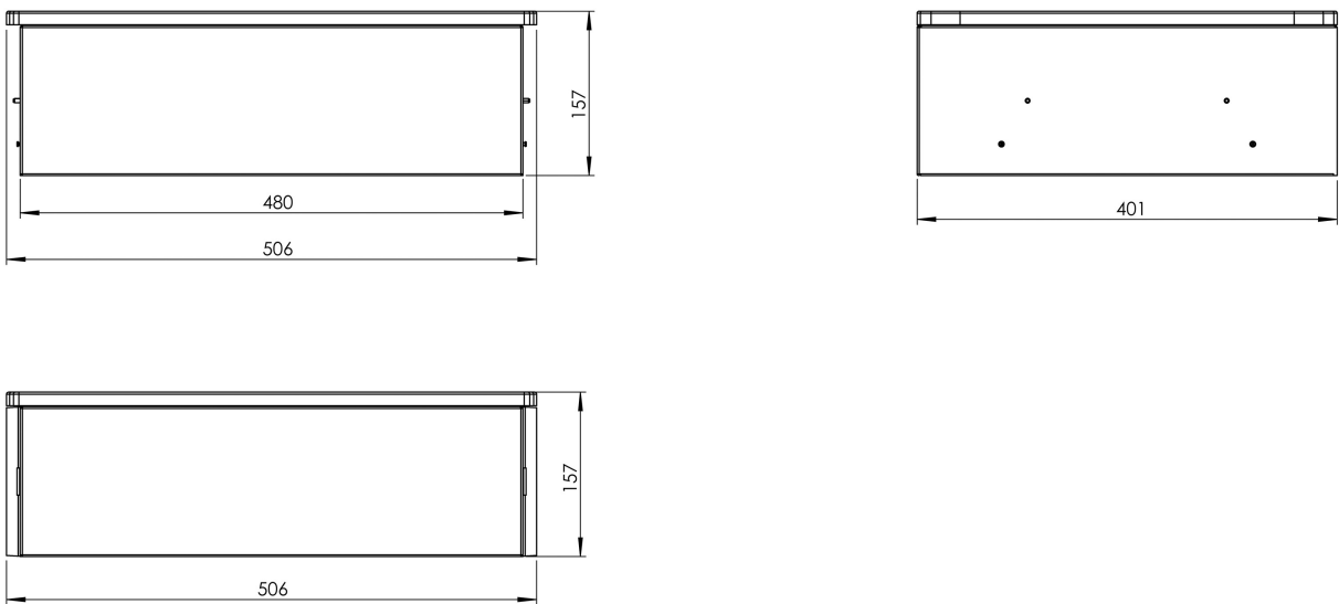
Abbildung 6. Abmessungen — Extension-Box
