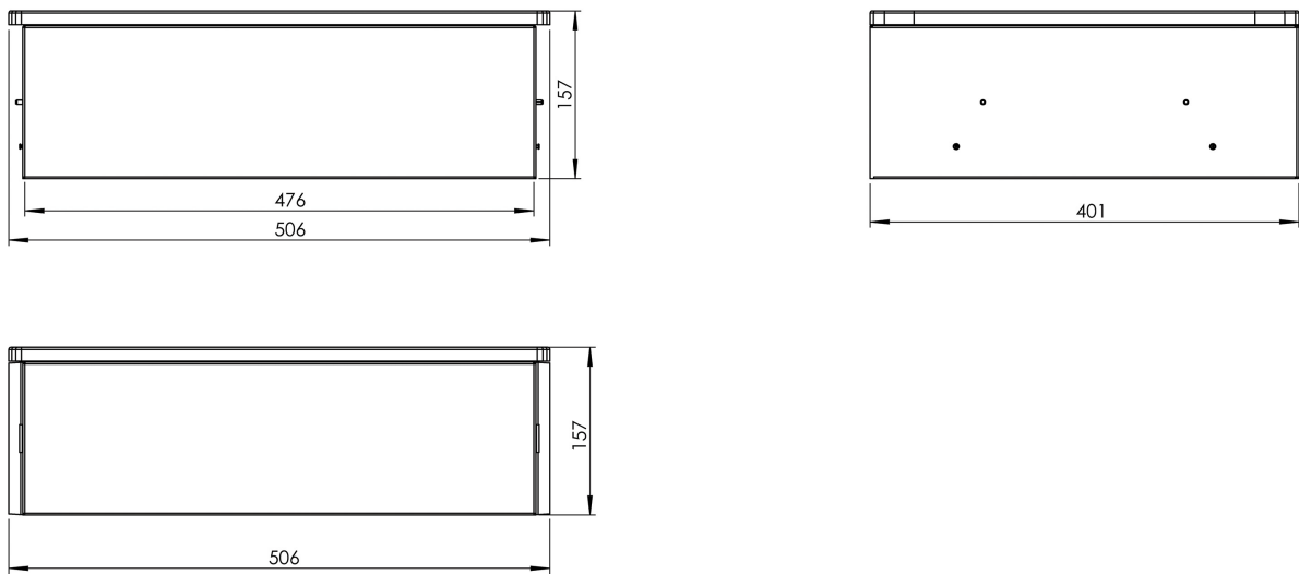
Abbildung 4. Abmessungen — Parallel-Box
