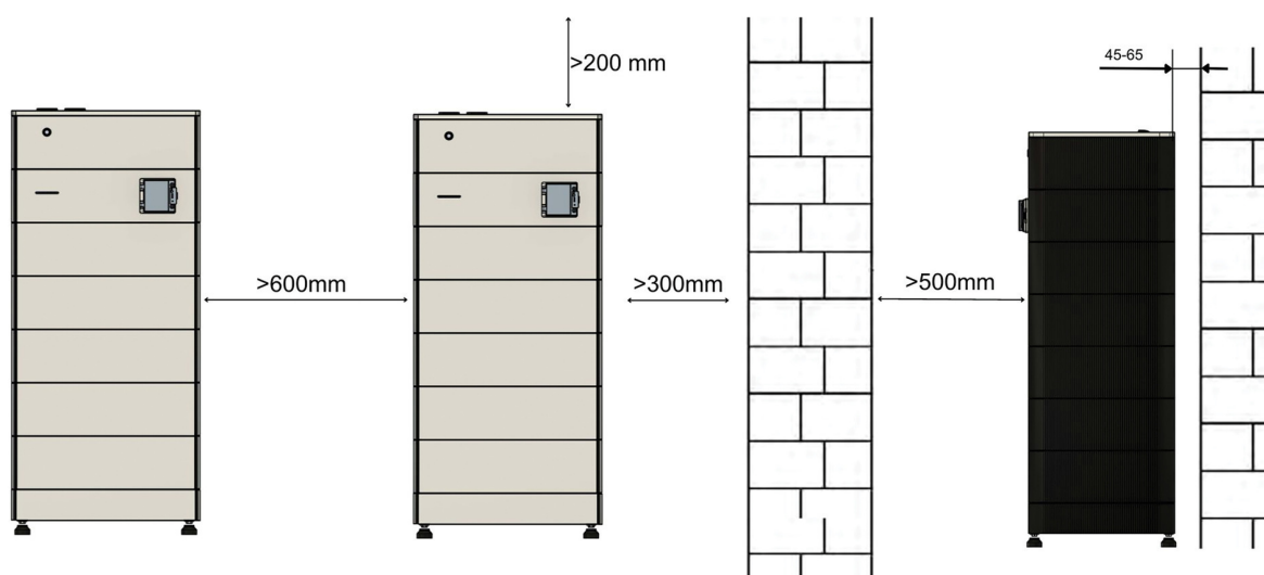
Abbildung 19. Abstände am Aufstellort
