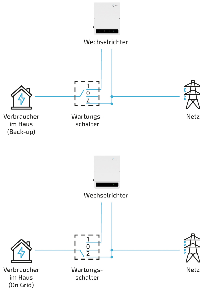
Abbildung 23. Empfohlener Wartungsschalter für Notstromabgang
