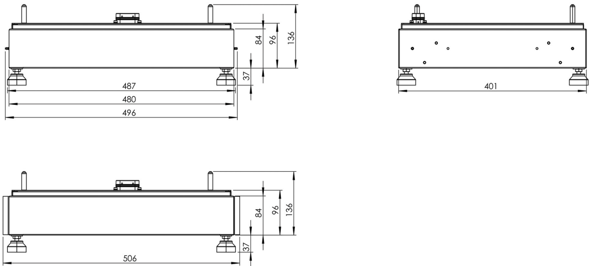
Abbildung 9. Abmessungen — Sockel
