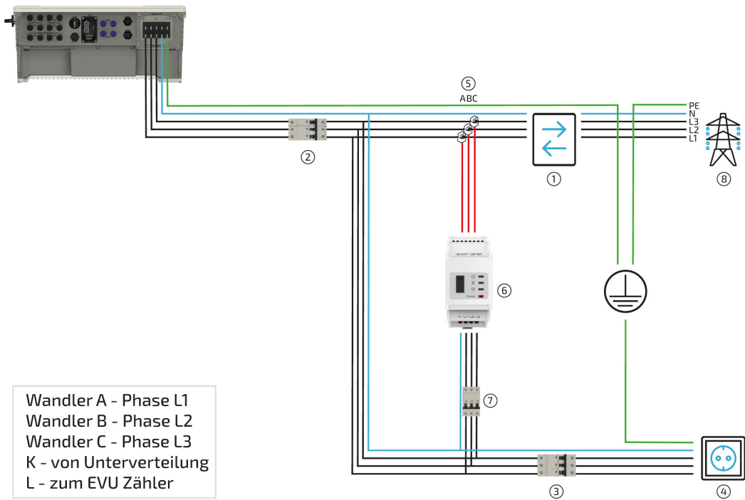
Abbildung 24. AC-Anschluss Energy-Meter
