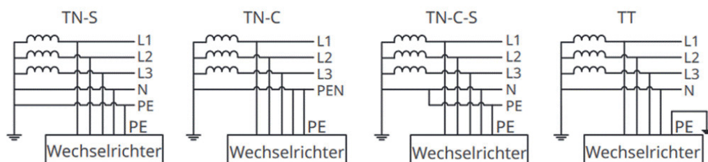
Abbildung 21. Zugelassen Netzformen für den Anschluss des FENECON Home 20 & 30
