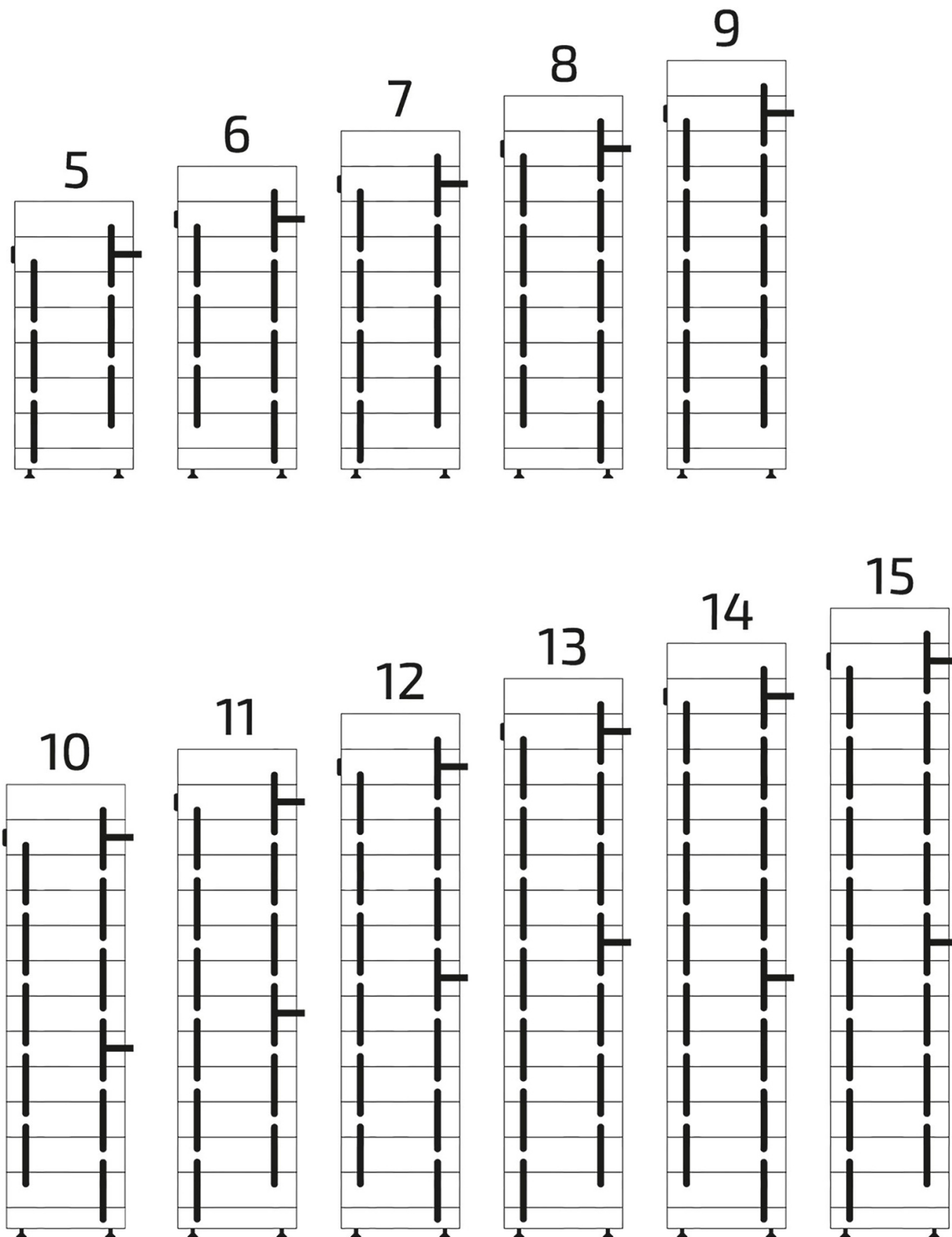
Abbildung 20. Anordnung der Modulbefestigung
