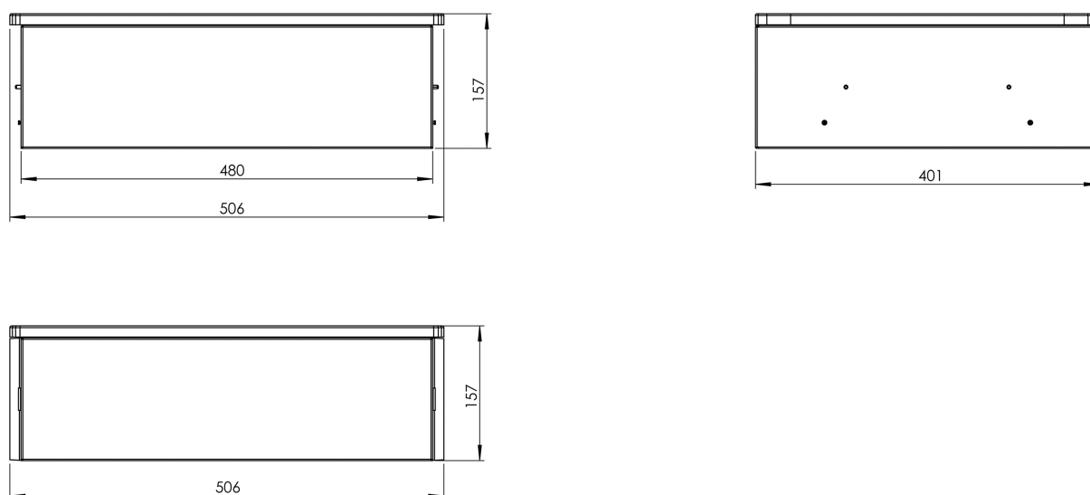
Abbildung 6. Abmessungen — Extension-Box
