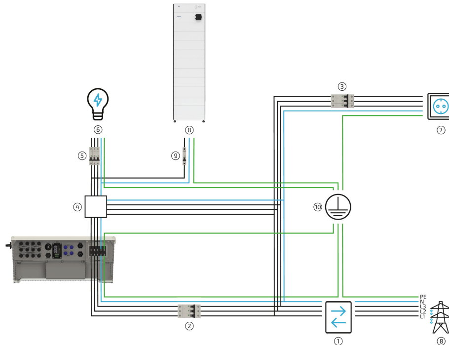
Abbildung 22. AC-Anschluss allgemein
