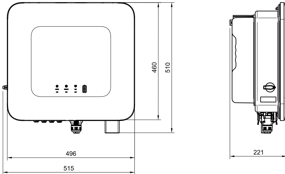
Abbildung 1. Abmessungen — Wechselrichter
