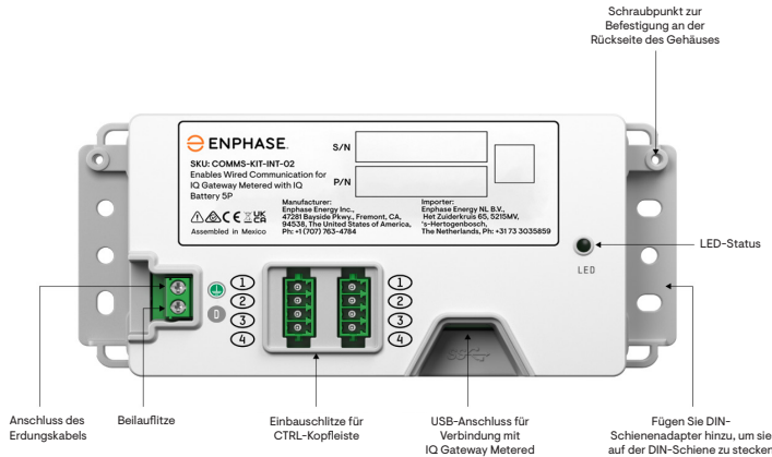
Abbildung 1: Vorderansicht von Communications Kit 2 INT
