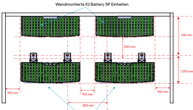
Wandmontierte IQ Battery 5P Einheiten
