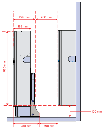
Mindestabstand vom Boden bis zur Unterseite des Geräts (sowohl bei Boden- als auch bei Wandmontage)
