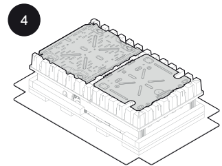
Die Schutzabdeckung oben und die Montagehalterung* unten entfernen
