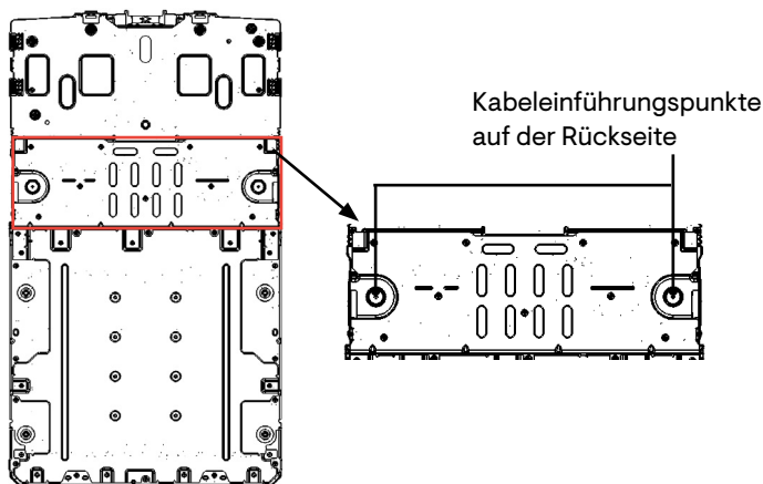
Kabeleinführungen auf der Rückseite der IQ Battery 5P
