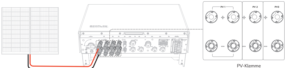
PV-Klemme
