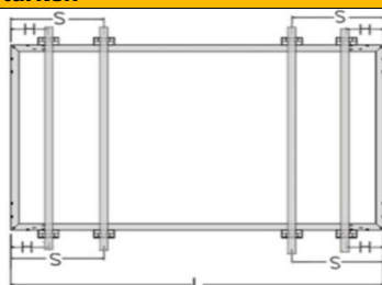
Abbildung 14 Klemme-I
