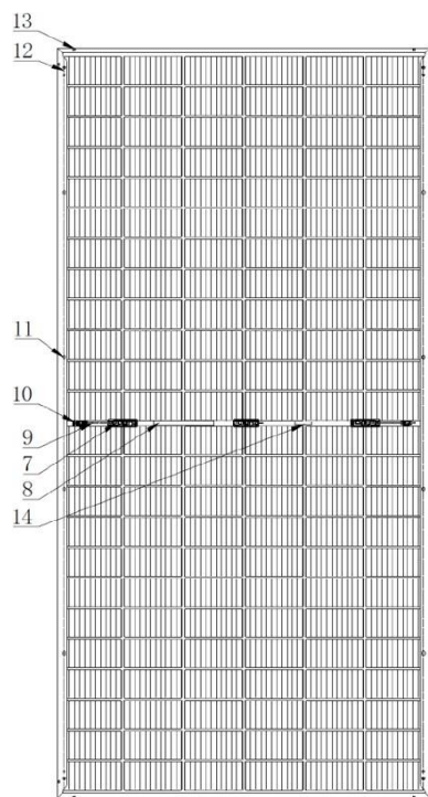
Aufbau von Doppelglasmodulen und Bauteilbezeichnung
