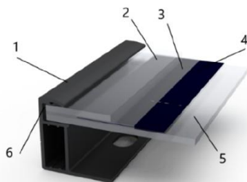
Aufbau von Doppelglasmodulen und Bauteilbezeichnung
